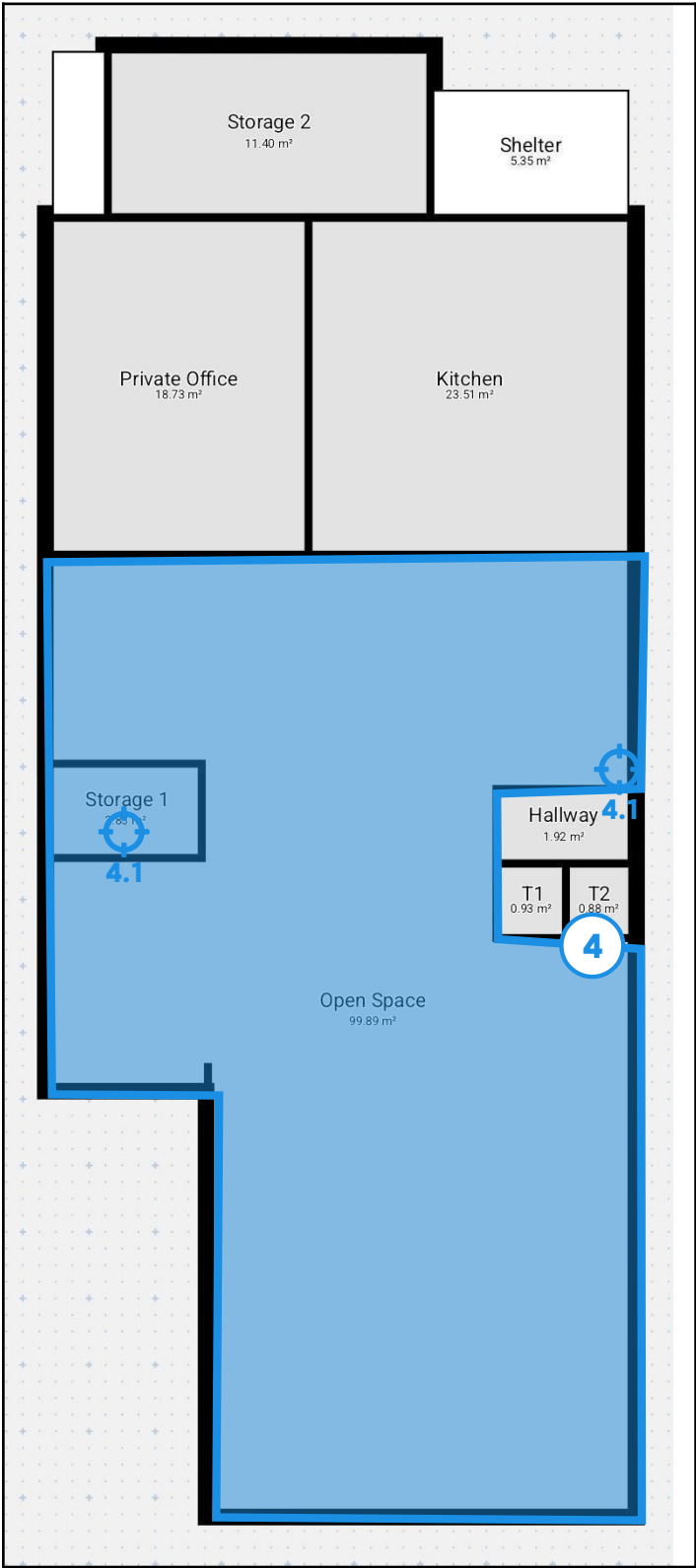
Legende van plan 1.4: Horecaruimte gelijkvloers
